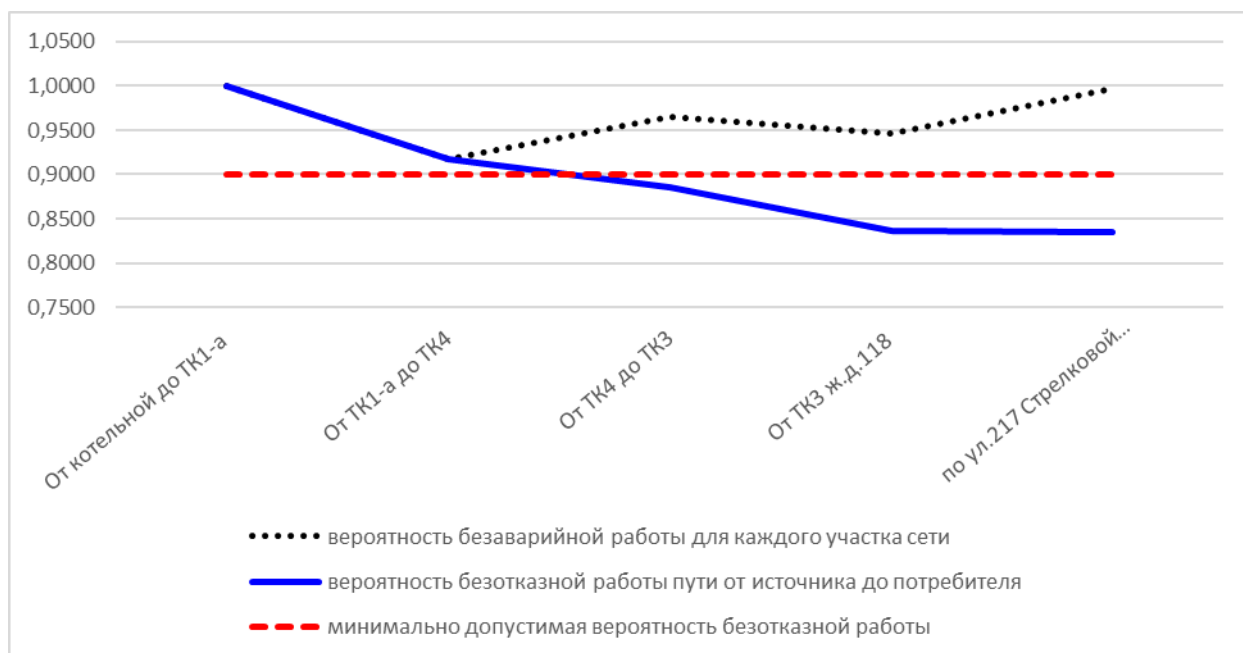
Рис. 11.3.14.1. Вероятность безаварийной работы теплосети от котельной №26 ул.Чкалова, 26-б до ж.д.118 по ул.217 Стрелковой дивизии
