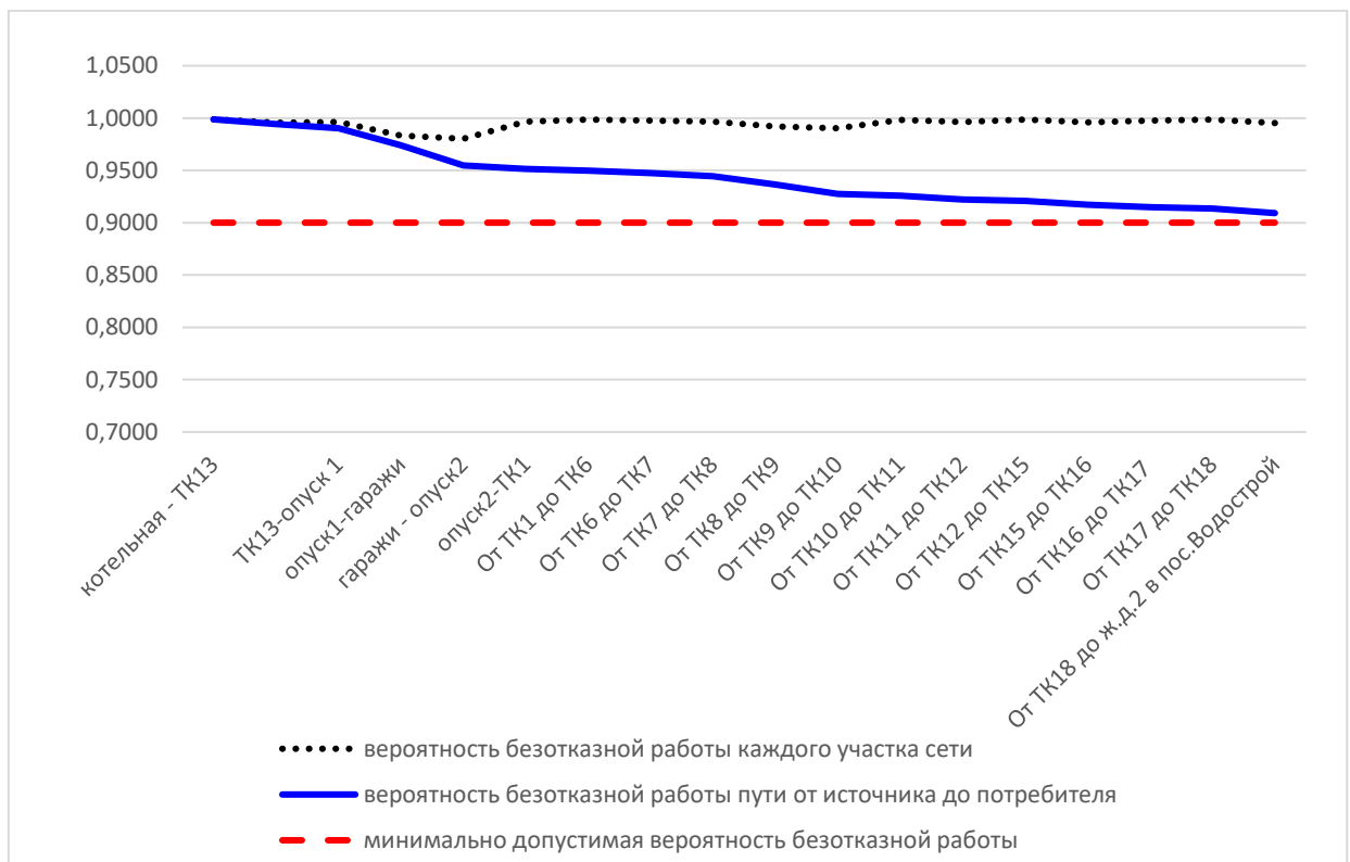
Рис. 11.3.19. Вероятность безаварийной работы теплосети от котельной пос.Водострой до ж.д.2 в пос.Водострой
