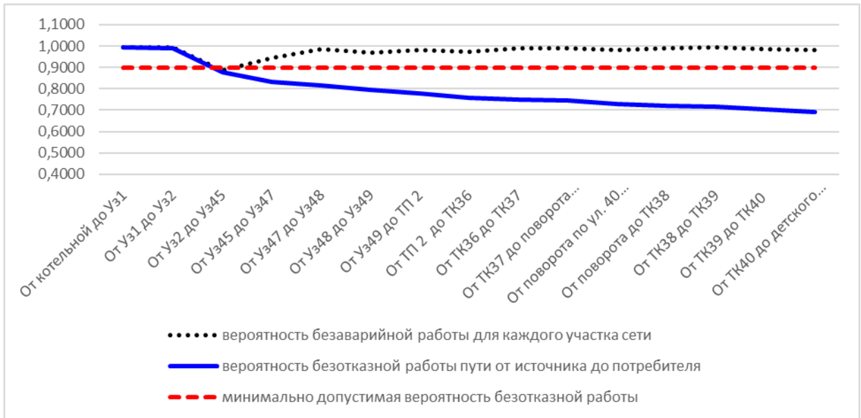
Рис. 11.3.22.2. Вероятность безаварийной работы теплосети от котельной ул. 40 лет Октября, 43 до детского сада №16
