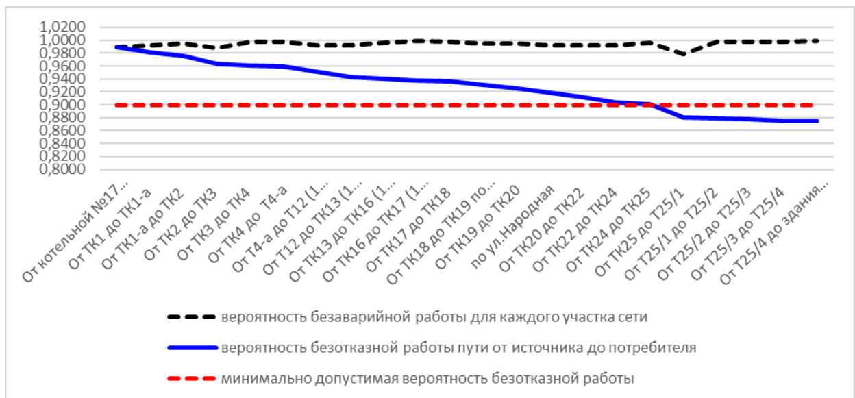
Рис. 11.3.9.1. Вероятность безаварийной работы теплосети от котельной №17 ул.Свободы, 207-а до здания 78 по ул.К.Маркса
