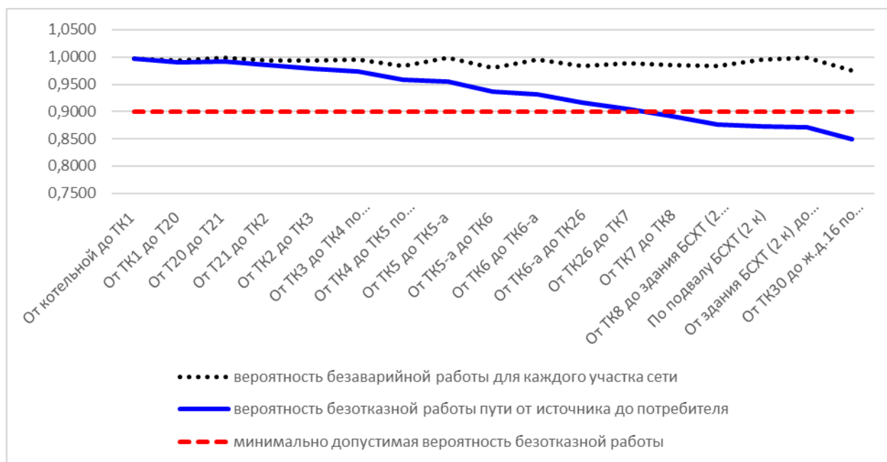
Рис. 11.3.16. Вероятность безаварийной работы теплосети от котельной №29 ул.Советская, 13-а до ж.д.16 по ул.Советская
