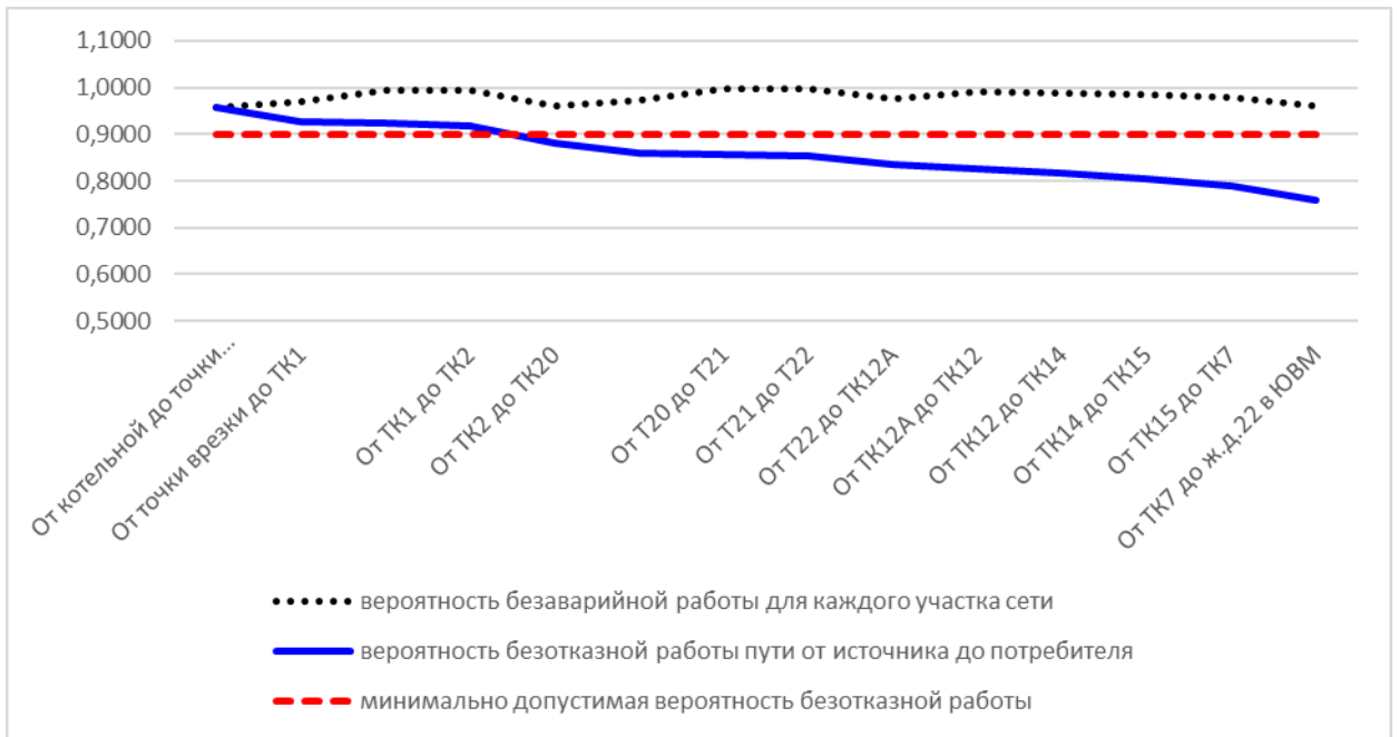
Рис. 11.3.23.2. Вероятность безаварийной работы теплосети от котельной ул. 40 лет Октября, 321 до ж.д.22 в ЮВМ
