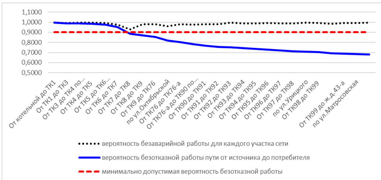
Рис. 11.3.3.2. Вероятность безаварийной работы теплосети от котельной №4 ул.Бланская, 109-б до ж.д.43-а по ул.Матросовская
