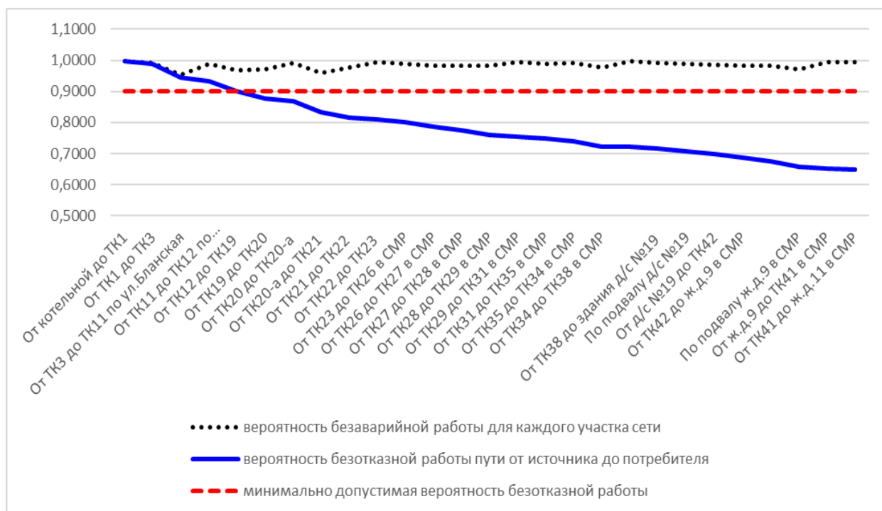
Рис. 11.3.3.1. Вероятность безаварийной работы теплосети от котельной №4 ул.Бланская, 109-б до ж.д.11 в Северном м-не
