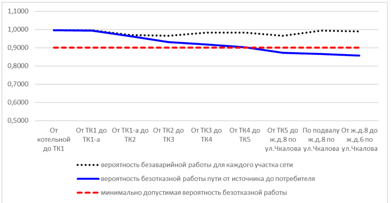
Рис. 11.3.24.2 Вероятность безаварийной работы теплосети от котельной ул. Чкалова, 1-е до ж.д.6 по ул.Чкалова
