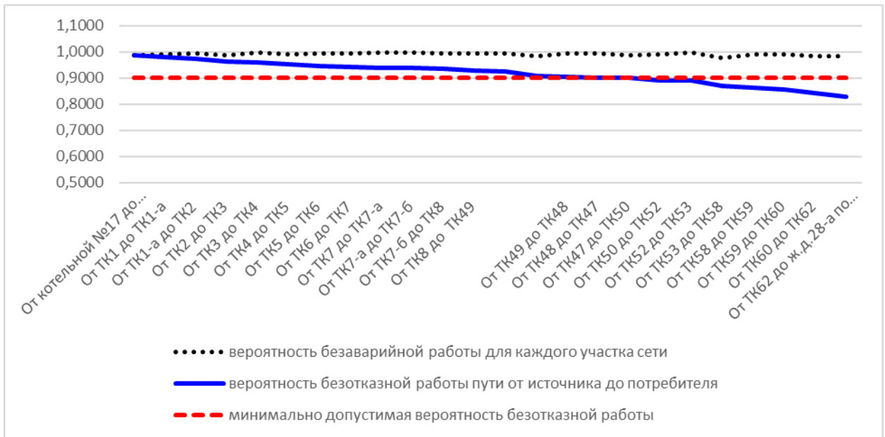
Рис. 11.3.9.2. Вероятность безаварийной работы теплосети от котельной №17 ул.Свободы, 207-а до ж.д.28-а по ул.Народная
