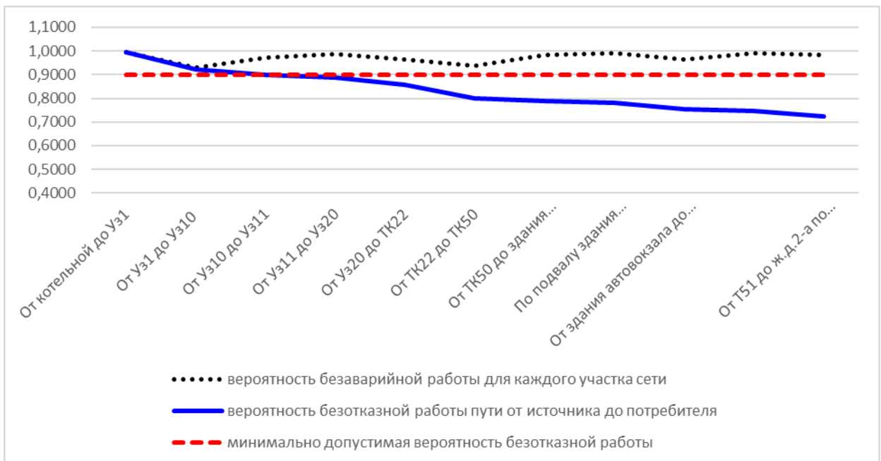
Рис. 11.3.22.2. Вероятность безаварийной работы теплосети от котельной ул. 40 лет Октября, 43 до ж.д.2-а по ул.Сенная
