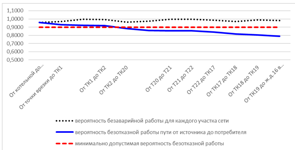
Рис. 11.3.23.1. Вероятность безаварийной работы теплосети от котельной ул. 40 лет Октября, 321 до ж.д.16 в ЮВМ
