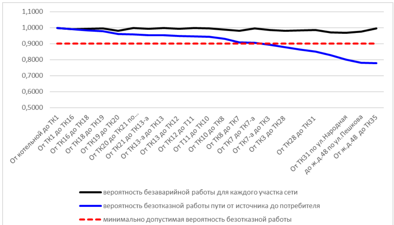
Рис. 11.3.1. Вероятность безаварийной работы теплосети от котельной №1 ул. Третьяковская, 14-а до ж.д.41-а по ул. Пешкова
