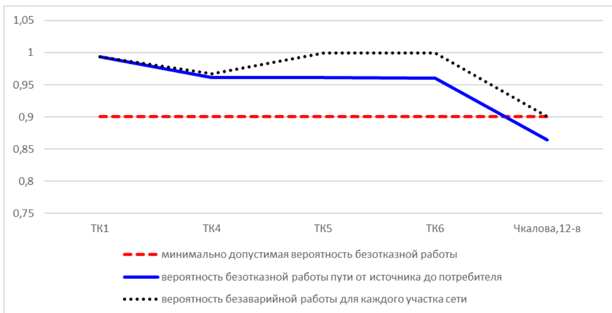
Рис. 11.3.2. Вероятность безаварийной работы теплосети от котельной №2 ул.Чкалова, 16-б до ж.д.12-в по ул.Чкалова
