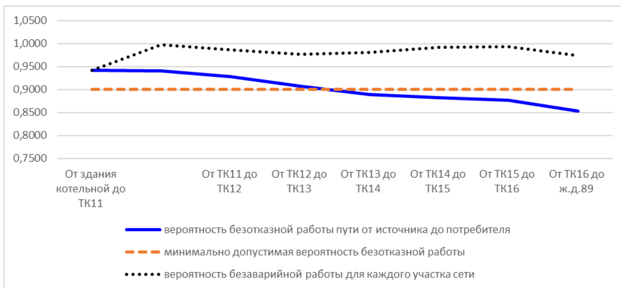
Рис. 11.3.10. Вероятность безаварийной работы теплосети от котельной №18 пер.Пушкинский, 8-б до ж.д.89 по ул.Пушкинская
