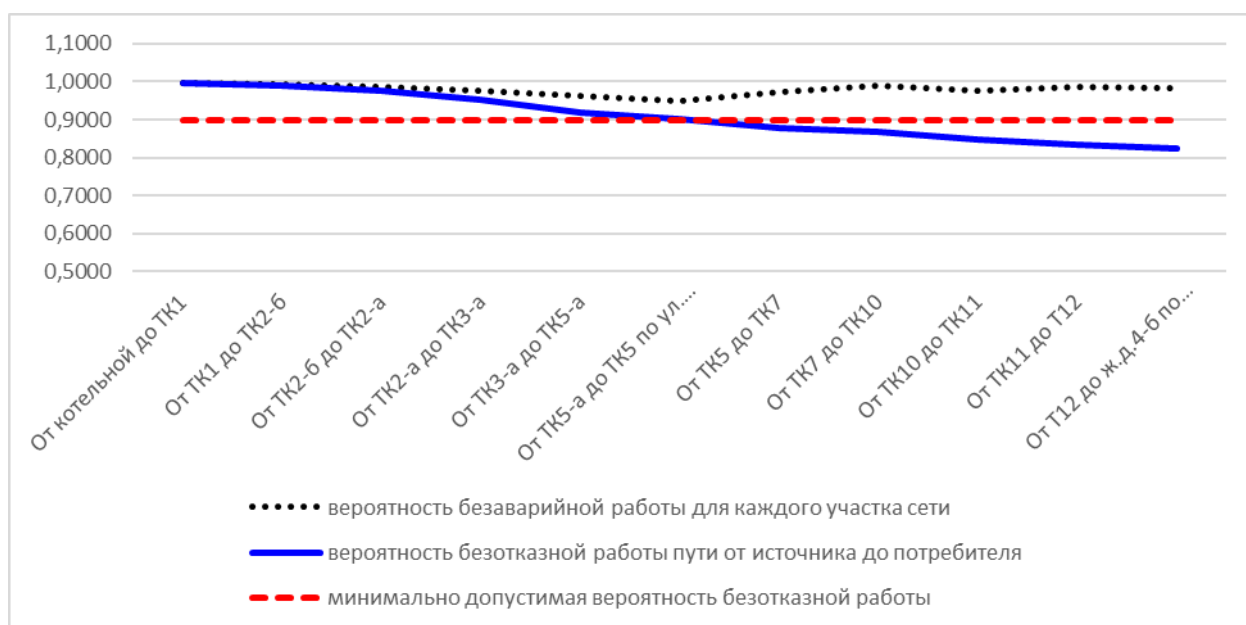
Рис. 11.3.24.1 Вероятность безаварийной работы теплосети от котельной ул. Чкалова, 1-е до ж.д.4-б по Поворинскому пр.
