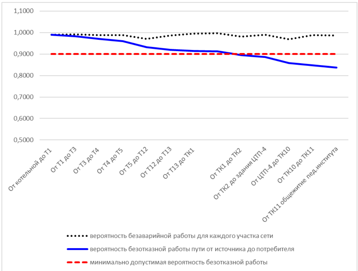
Рис. 11.3.20.1. Вероятность безаварийной работы теплосети от котельной ОАО "Патроны" ул.Бланская, 69 до общежития пед.института ул Советская, 11
