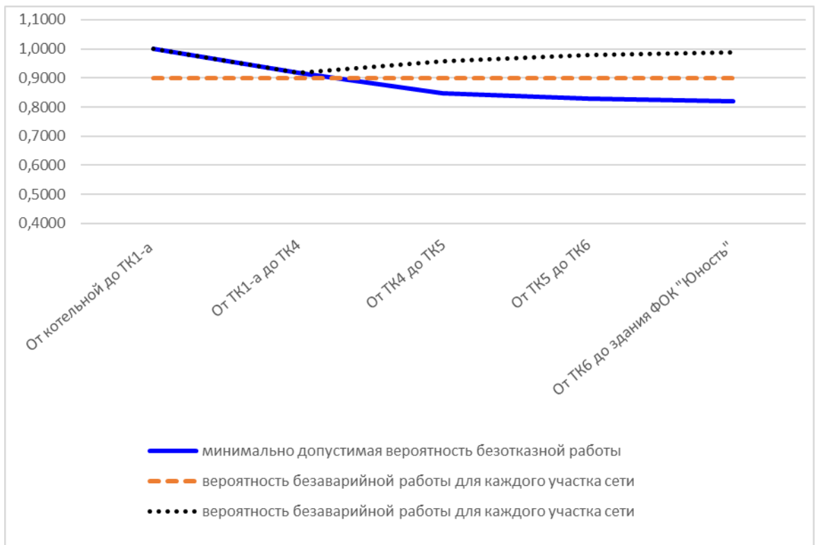
Рис. 11.3.14.1. Вероятность безаварийной работы теплосети от котельной №26 ул. Чкалова, 26-б до ФОК "Юность"
