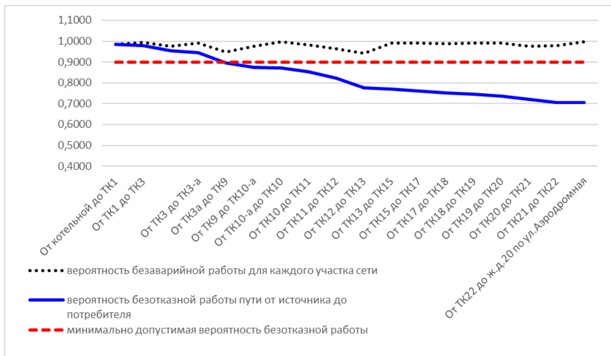
Рис. 11.3.21.1. Вероятность безаварийной работы теплосети от котельной ул.Советская, 82-а до ж.д.20 по ул.Аэродромная
