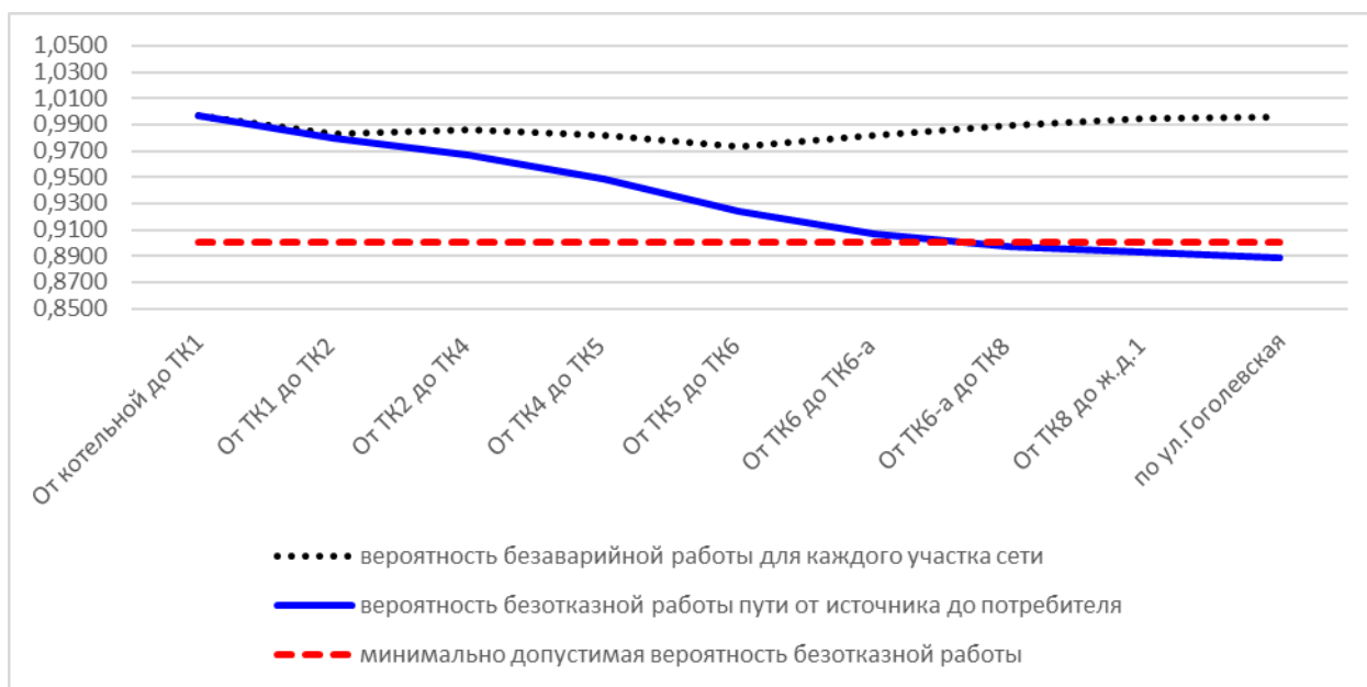
Рис. 11.3.4. Вероятность безаварийной работы теплосети от котельной №5 ул.Гоголевская, 14-б до ж.д.1 по ул.Гоголевская
