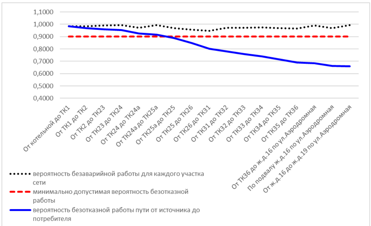
Рис. 11.3.21.2. Вероятность безаварийной работы теплосети от котельной ул.Советская, 82-а до ж.д.19 по ул.Аэродромная
