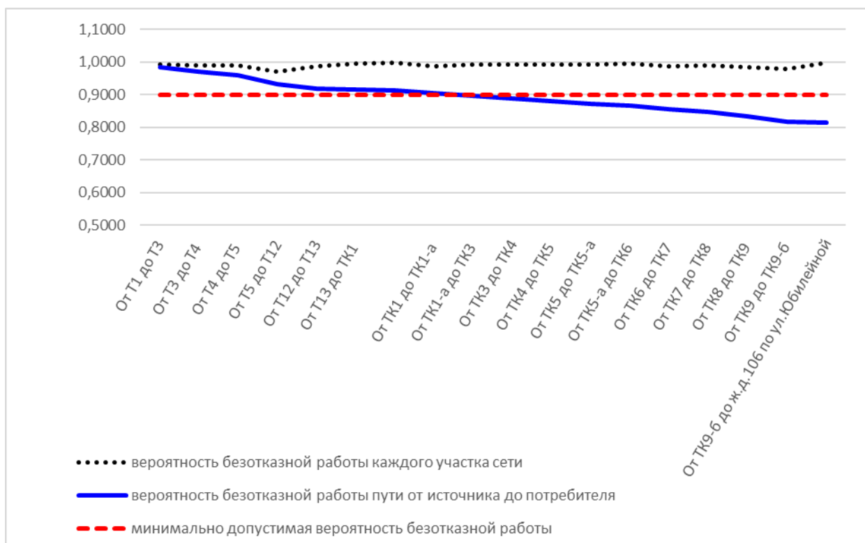
Рис. 11.3.20.1. Вероятность безаварийной работы теплосети от котельной ОАО "Патроны" ул.Бланская, 69 до ж.д.106 по ул.Юбилейной
