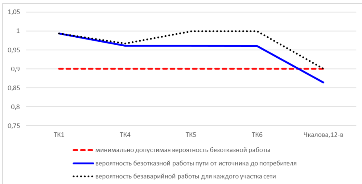
Рис. 11.3.2. Вероятность безаварийной работы теплосети от котельной №2 ул.Чкалова, 16-б до ж.д.12-в по ул.Чкалова
