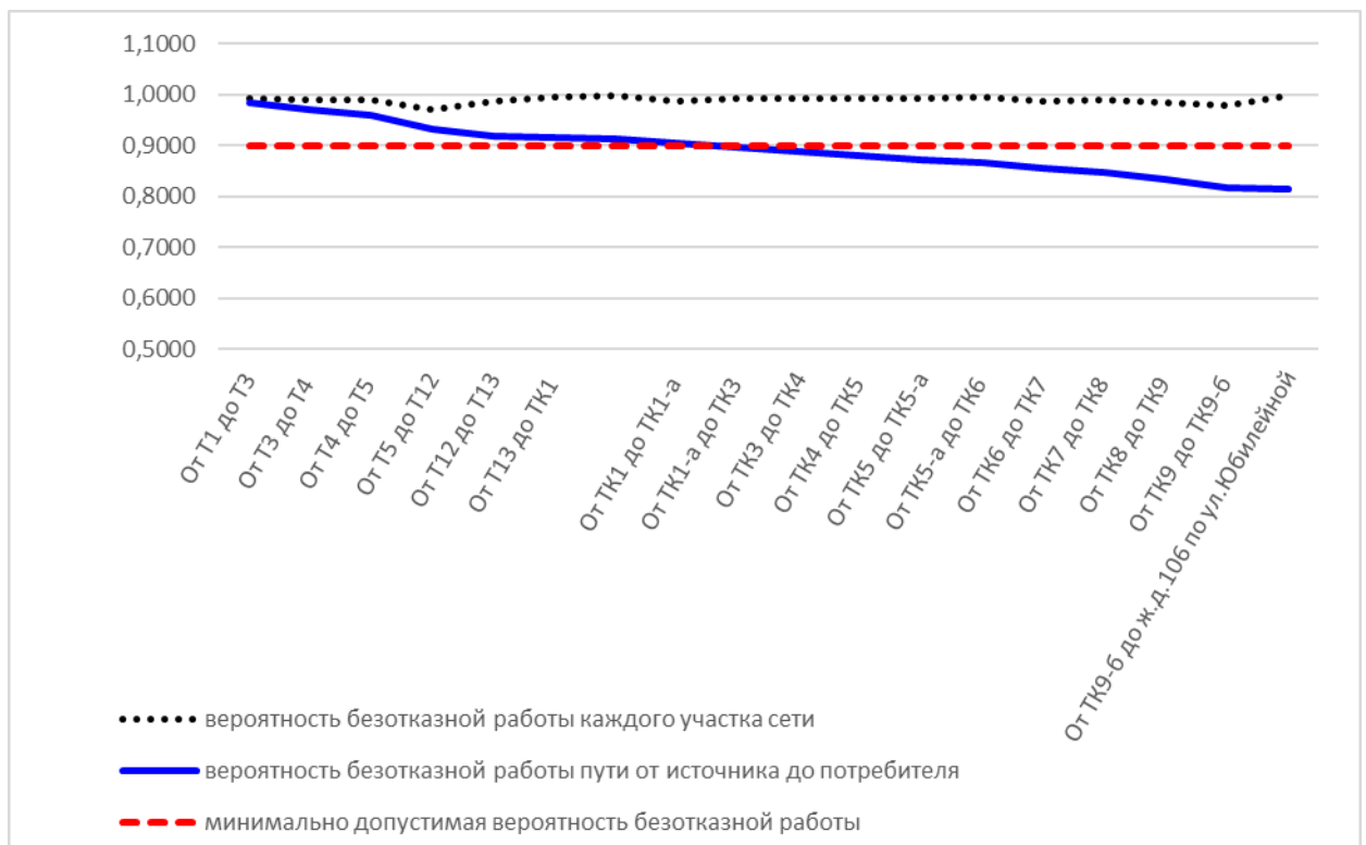
Рис. 11.3.20.1. Вероятность безаварийной работы теплосети от котельной ОАО "Патроны" ул.Бланская, 69 до ж.д.106 по ул.Юбилейной
