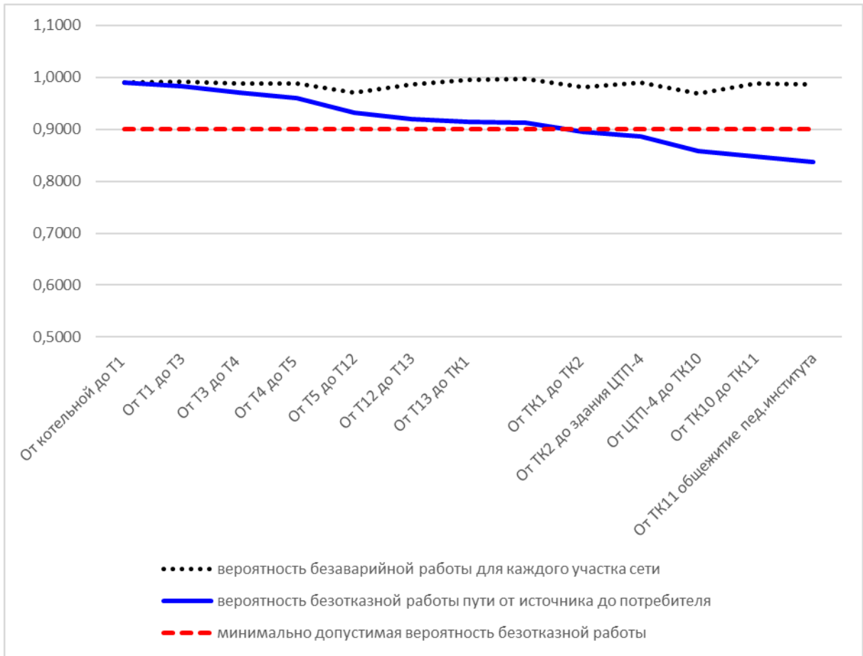
Рис. 11.3.20.1. Вероятность безаварийной работы теплосети от котельной ОАО "Патроны" ул.Бланская, 69 до общежития пед.института ул Советская, 11
